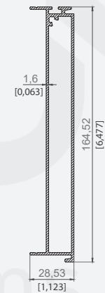
DERE UZATMA PROFİLİ GUTTER EXTENTION PROFILE
