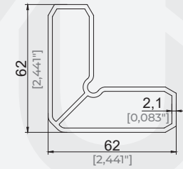
KASA KÖŞE TAKOĞU PROFİLİ FRAME CORNER WEDGE PROFILE
