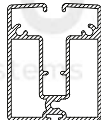
2937 Saçak Profili Fringe Profile
