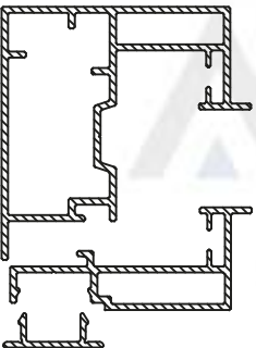
2877 Dikme Profili Sewing Profile
